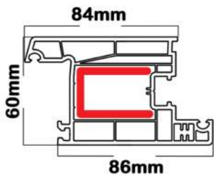
Door Sash profile
