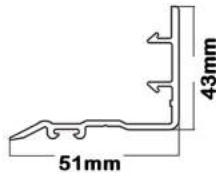
Sliding door interlock
