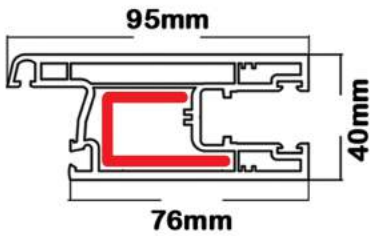
Sliding door sash Profile
